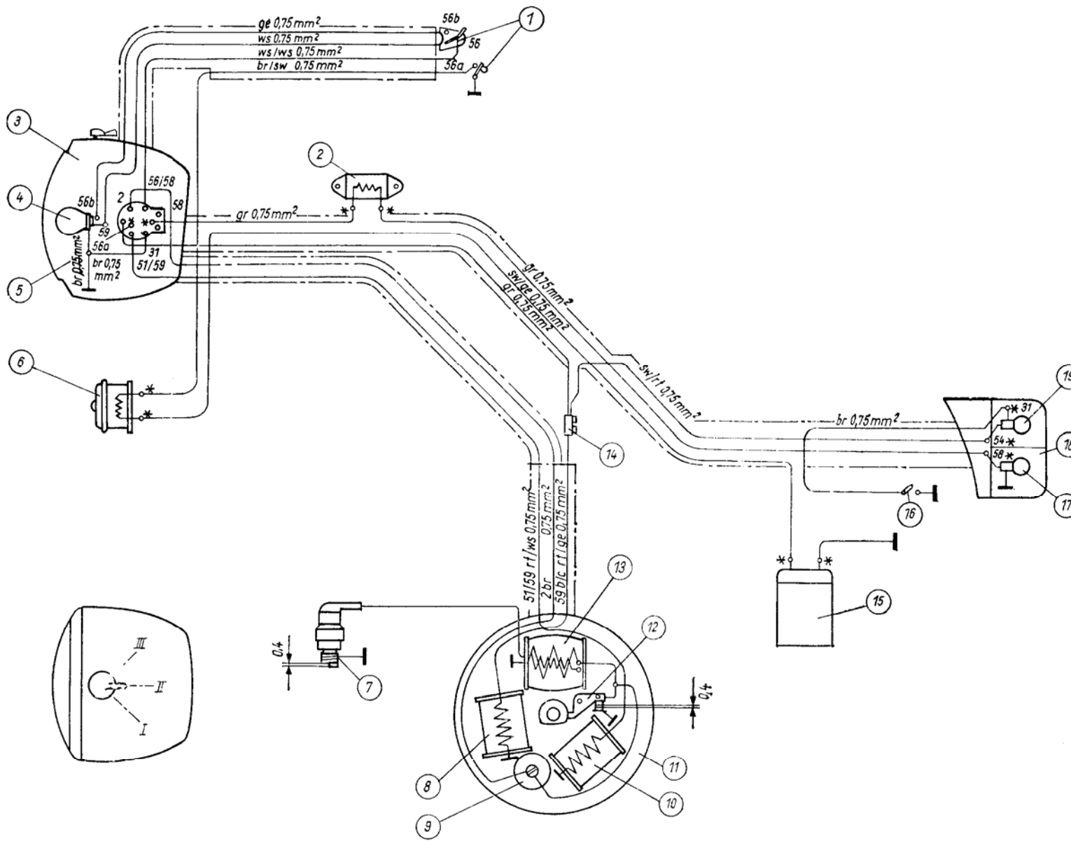
Bild 246. Schaltplan für SR 4-1
